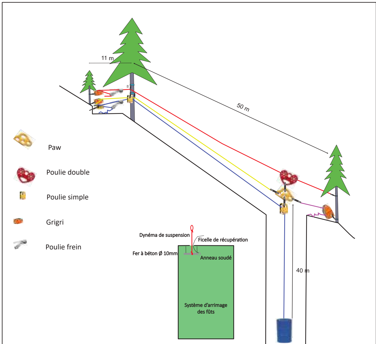
Figure 1 - Schéma de principe du système d'évacuation des fûts
